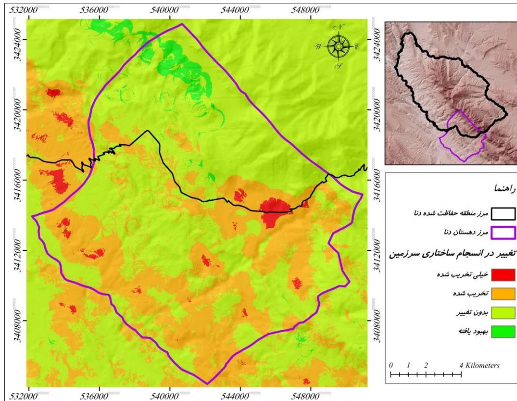
شکل ۴. طبقات تغییرات انسجام ساختاری سرزمین (در مناطق قرمز رنگ، بیشترین کاهش انسجام ساختاری بر اساس پوشش جنگل رخ داده است و در مناطق سبز پررنگ برعکس)
