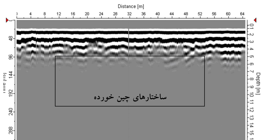
شکل شماره ۸. نیمرخ اول رادارسراب یآوری (تفسیرها بر اساس تغییرات موج و شکل آنها صورت گرفته است)
