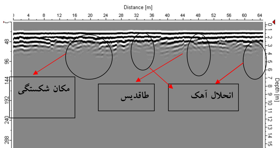
شکل ۷. نیمرخ اول رادارسراب یآوری (تفسیرها بر اساس تغییرات موج و شکل آنها صورت گرفته است)
