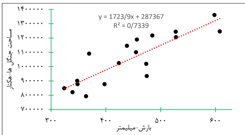
شکل ۸. پراکنش نگار ارتباط بین مساحت پهنه دارای پوشش سبزیگی بلوط‌های لرستان (شهریورماه) و مجموع بارش سالانه
