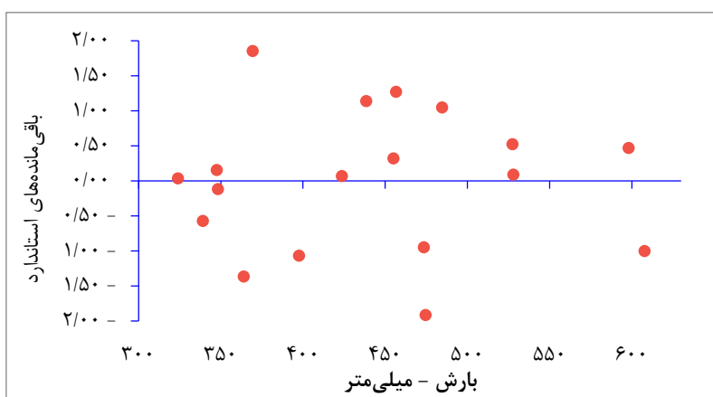
شکل ۷. باقی‌مانده‌های استاندارد شده مدل برازش داده شده بین مجموع بارش سالانه و پهنه پوشش جنگلی دارای آستانه تعیین شده سبزیگی جنگلی ( EVI > 0.4 )
