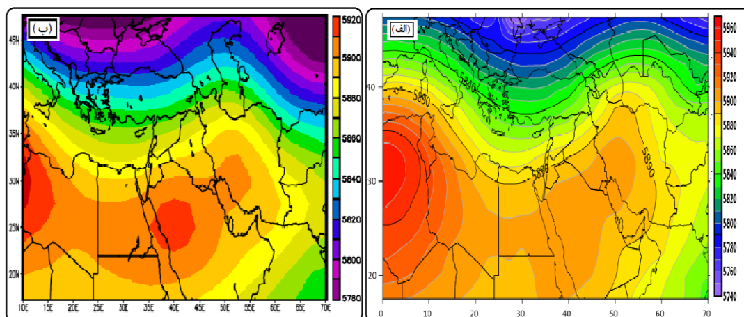
شکل ۲. نقشه میانگین ارتفاع ژئوپتانسیل تراز ۵۰۰ هکتوپاسکال در دوره پایه (الف)، و دوره اعمال محدودیت‌های کرونایی (ب).
