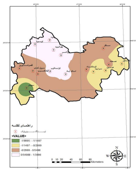
شکل ۶. تحلیل مکانی عامل دوم (جهت باد - بارش)
