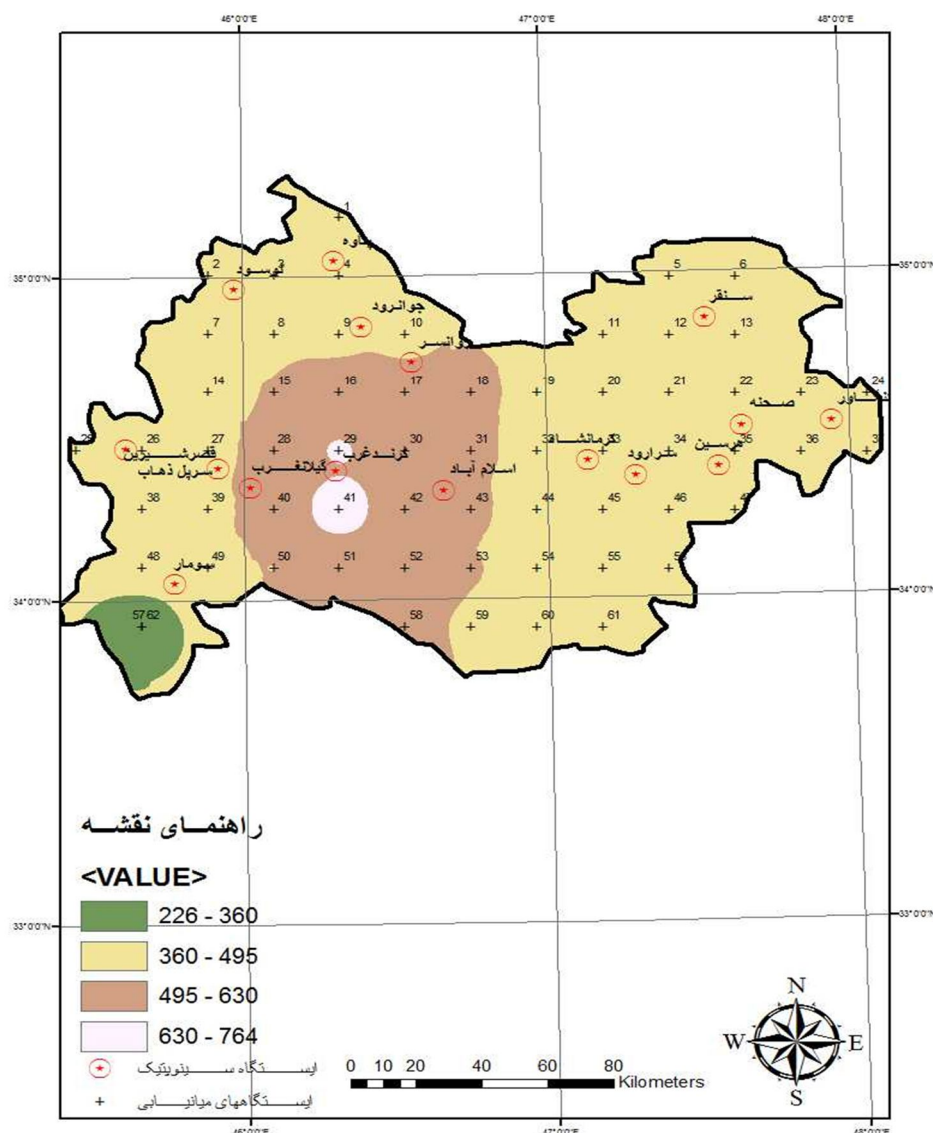
شکل ۲. نمونه‌ی فرایند میانابیی، عنصر اقلیمی بارش سالانه
