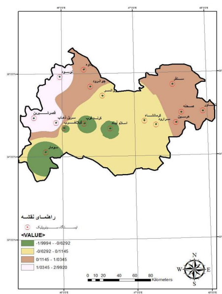
شکل ۷. تحلیل مکانی عامل سوم (رطوبت)
