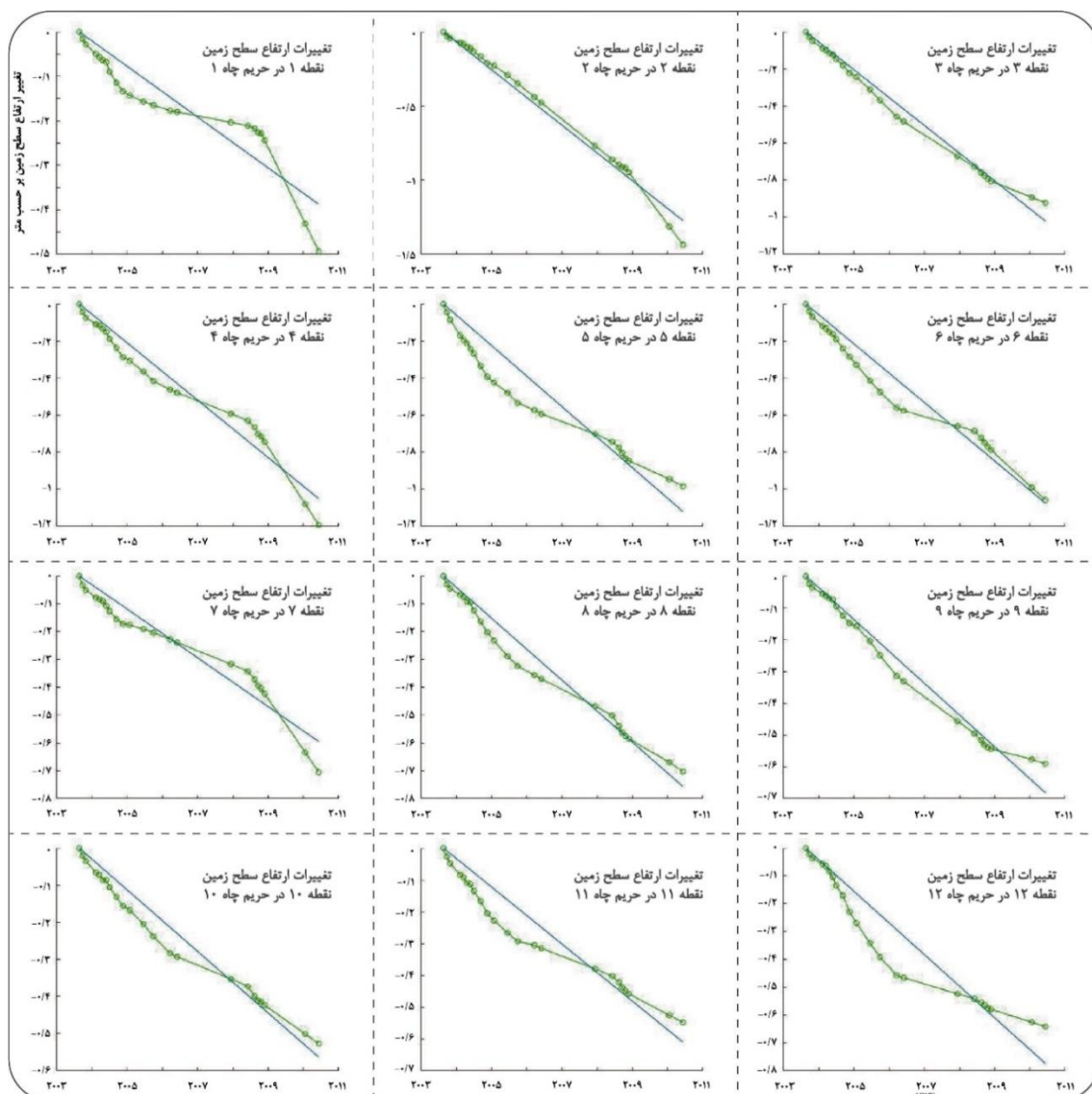
شکل ۴. تغییرات ارتفاع سطح زمین در حريم دوازده چاهک مشاهداتی - نقاط و خطوط منحنی نشان‌دهنده ارتفاع سطح زمین اندازه‌گیری شده به وسیله پردازش تداخل سنجی راداری و خط مستقیم رگرسیون آن است. (بازه زمانی ۲۰۰۳/۷/۱۸ تا ۲۰۱۰/۵/۷)
