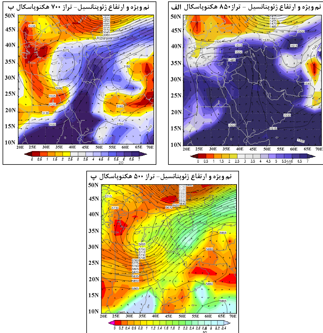
شکل ۱۳. توزیع نم و بژه (به گرم در هزار) و ارتفاع ژئوپتانسیل (به ژئوپتانسیل متر) ۲۹ اکتبر ۲۰۱۵: الف: تراز ۸۵۰ هکتوپاسکال؛ ب: تراز ۷۰۰ هکتوپاسکال و پ: ۵۰۰ هکتوپاسکال (خروجی Grads)
