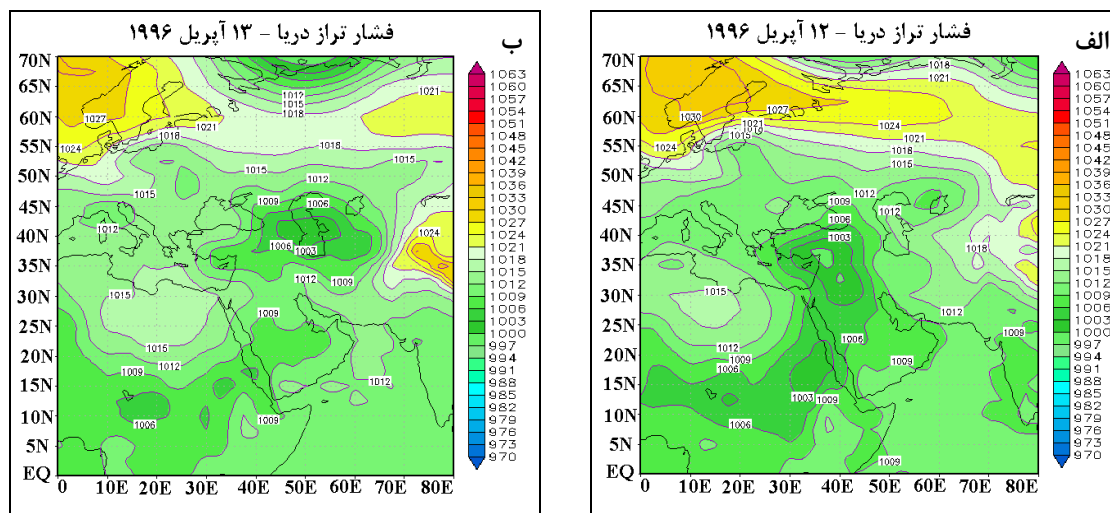
شکل ۸. نقشه فشار تراز دریا (به هکتوپاسکال) الف: در روزهای ۱۲ آوریل و ب: ۱۳ آوریل ۱۹۹۶ (خروجی Grads)
