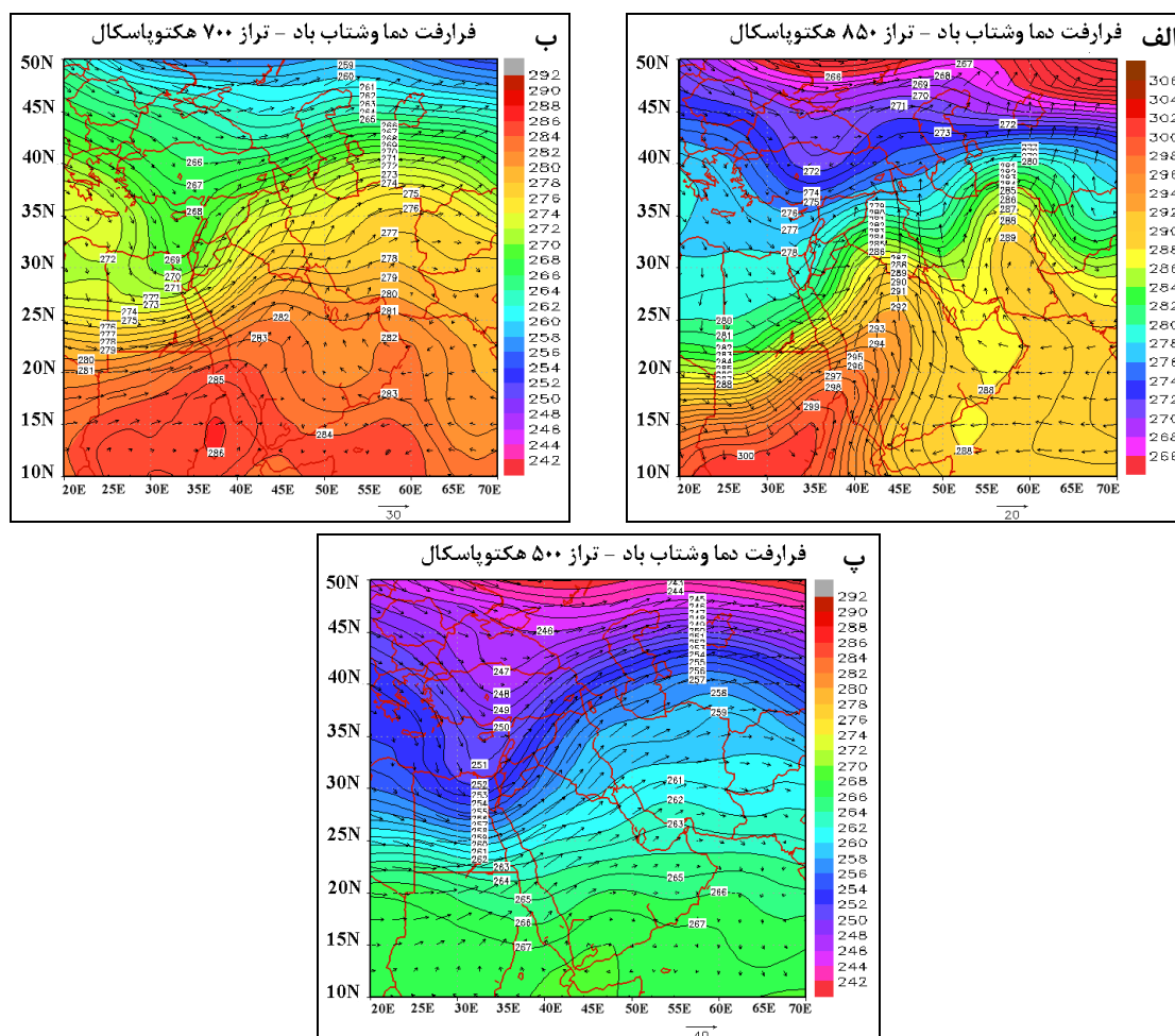
شکل ۶. وزش دمایی هوا (به درجه کلون)، الف: ۳ فوریه ۲۰۰۶؛ تراز ۸۵۰ هکتوپاسکال؛ ب: تراز ۷۰۰ هکتوپاسکال و پ: تراز ۵۰۰ هکتوپاسکال (خروجی Grads)
