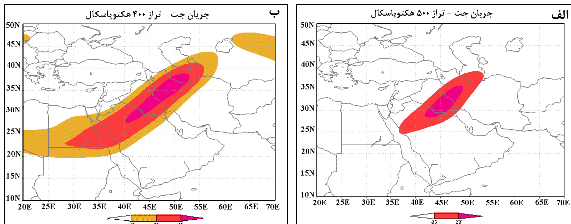
شکل ۱۱. جریان جت، الف: ۱۳ آوریل ۱۹۹۶؛ تراز ۵۰۰ هکتوپاسکال و ب: تراز ۴۰۰ هکتوپاسکال (خروجی Grads)
