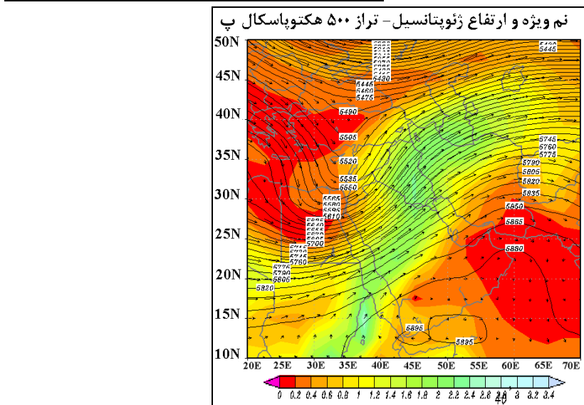
شکل ۵. توزیع نم و ویژه و ارتفاع ژئوپتانسیل (به ژئوپتانسیل متر)، الف: ۳ فوریه ۲۰۰۶؛ ب: تراز ۸۵۰ هکتوپاسکال؛ ب: تراز ۷۰۰ هکتوپاسکال و پ: ۵۰۰ هکتوپاسکال (خروجی Grads)
