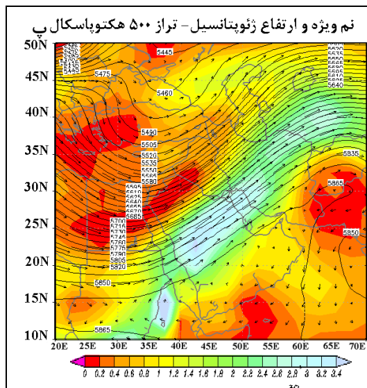
شکل ۹. توزیع نم و بزه و ارتفاع ژئوپتانسیل (به ژئوپتانسیل متر)، الف: ۱۳ آوریل ۱۹۹۶؛ تراز ۸۵۰ هکتوپاسکال؛ ب: تراز ۷۰۰ هکتوپاسکال و پ: ۵۰۰ هکتوپاسکال (خروجی Grads)
