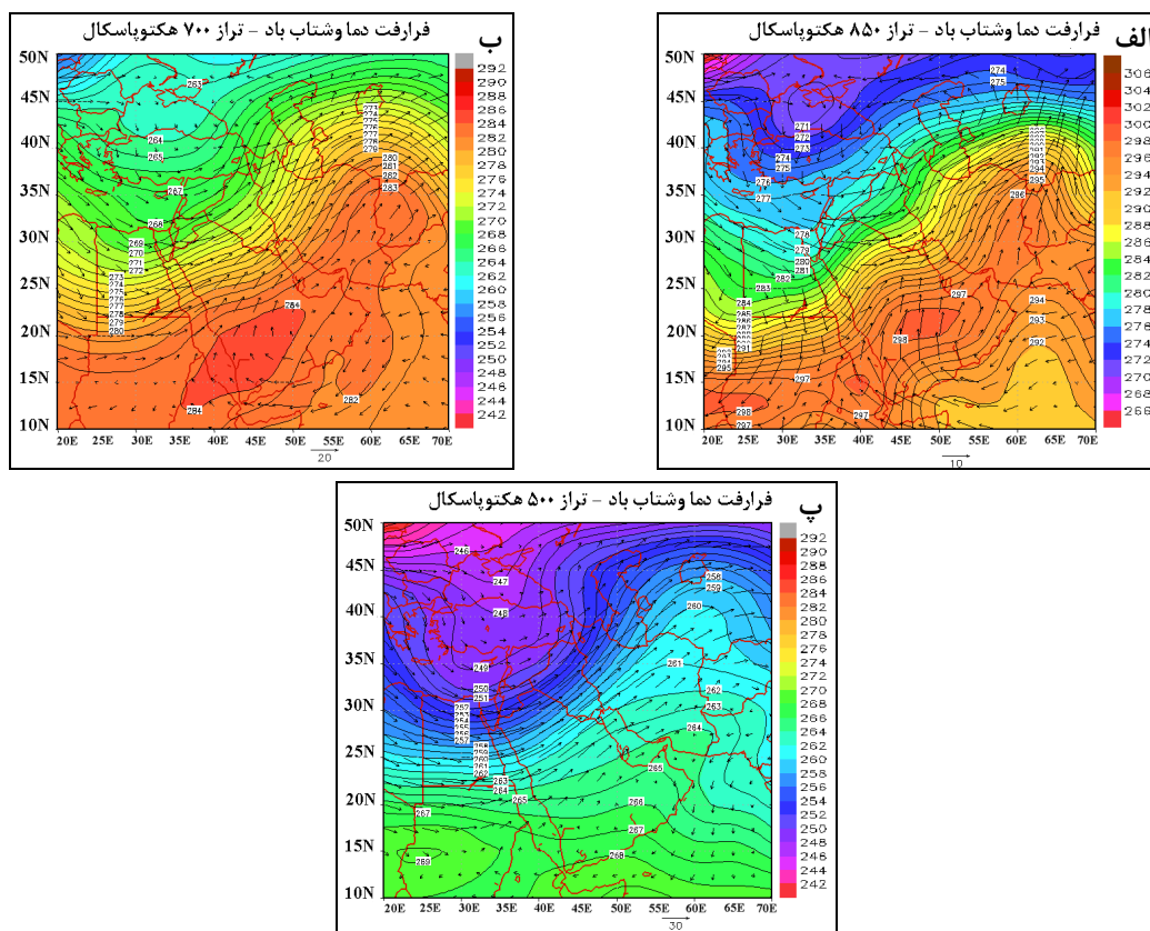
شکل ۱۰. وزش دمایی هوا (به درجه کلونین)، الف: ۱۳ آوریل ۱۹۹۶؛ تراز ۸۵۰ هکتوپاسکال؛ ب: تراز ۷۰۰ هکتوپاسکال و پ: ۵۰۰ هکتوپاسکال (خروجی Grads)
