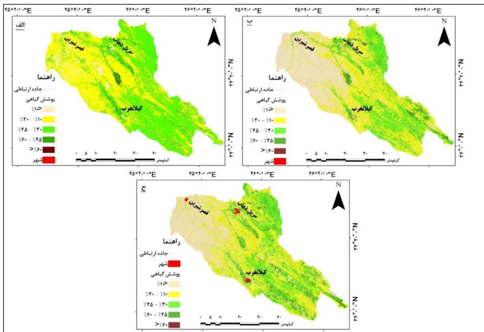
شکل ۳. نقشه پوشش گیاهی حوضه الوند؛ الف: سال ۲۰۱۸؛ ب: ۲۰۰۵؛ ج: ۱۹۹۰
