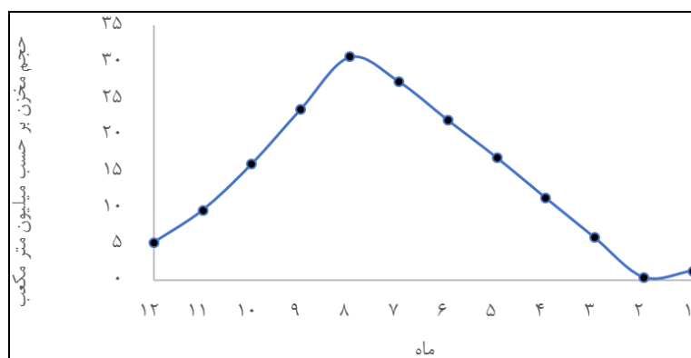
شکل ۳. منحنی فرمان سد مخزنی بیستون
