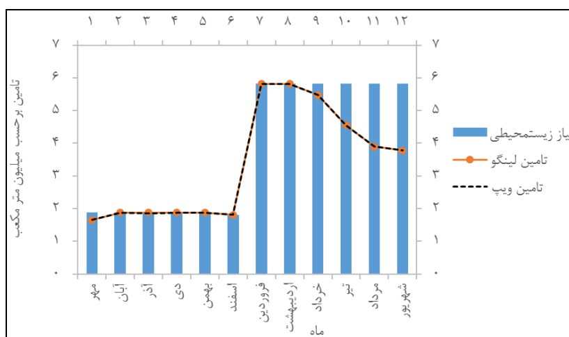
شکل ۶. مقایسه تأمین نیاز زیست‌محیطی بدون در نظر گرفتن سدهای بالادست رودخانه گاماسیاب
